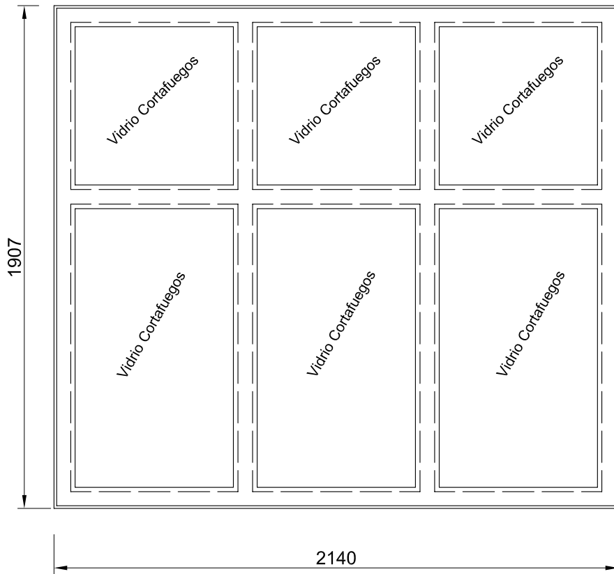
ALZADO
