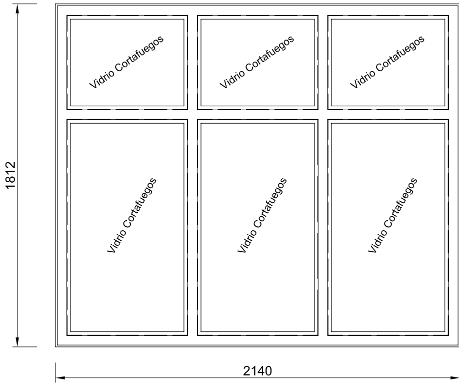
ALZADO
